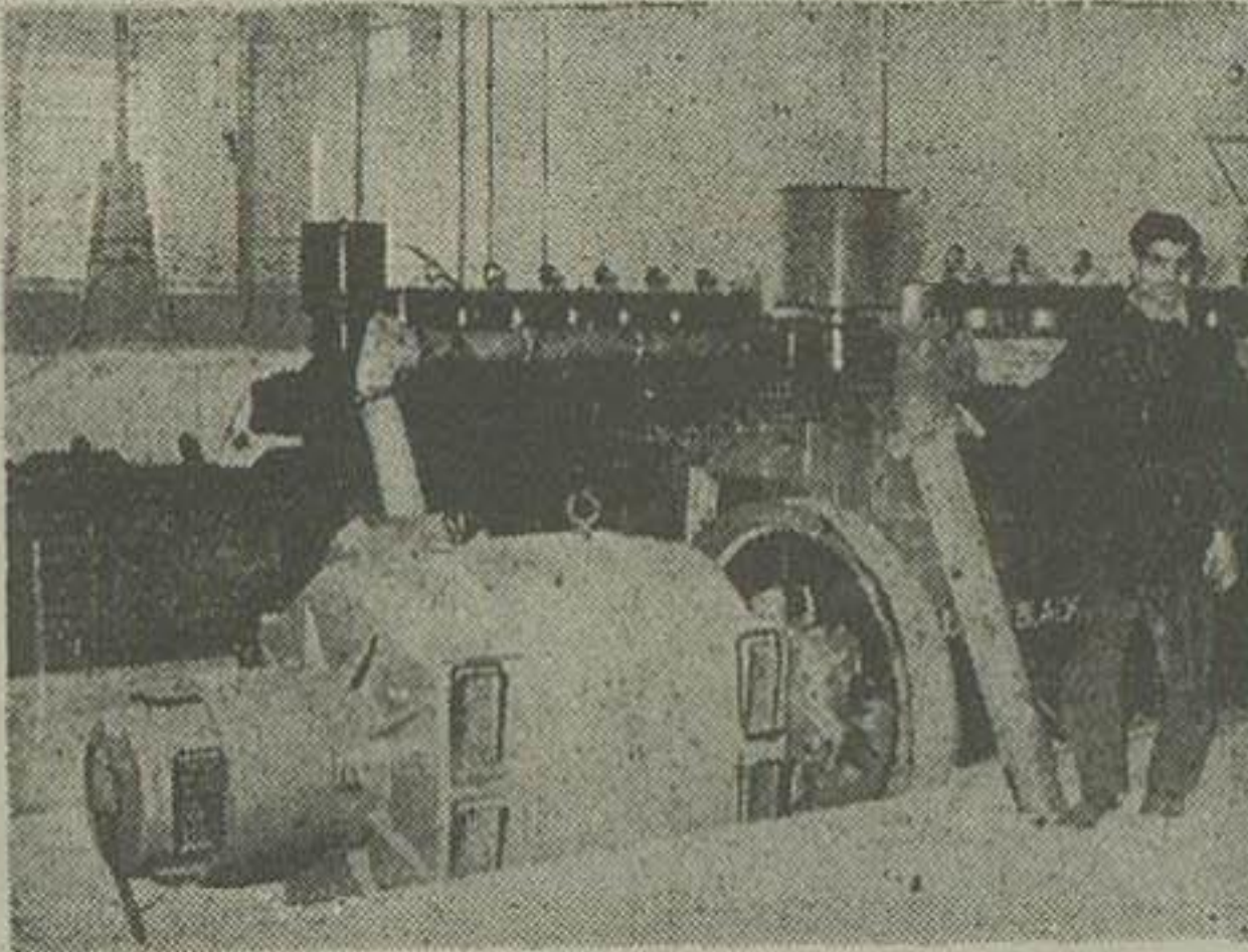
یک قسمت از موتورخانه برق «تهران پارس» که فعلاً در حدود هزار کیلوات برق تولید می کند
