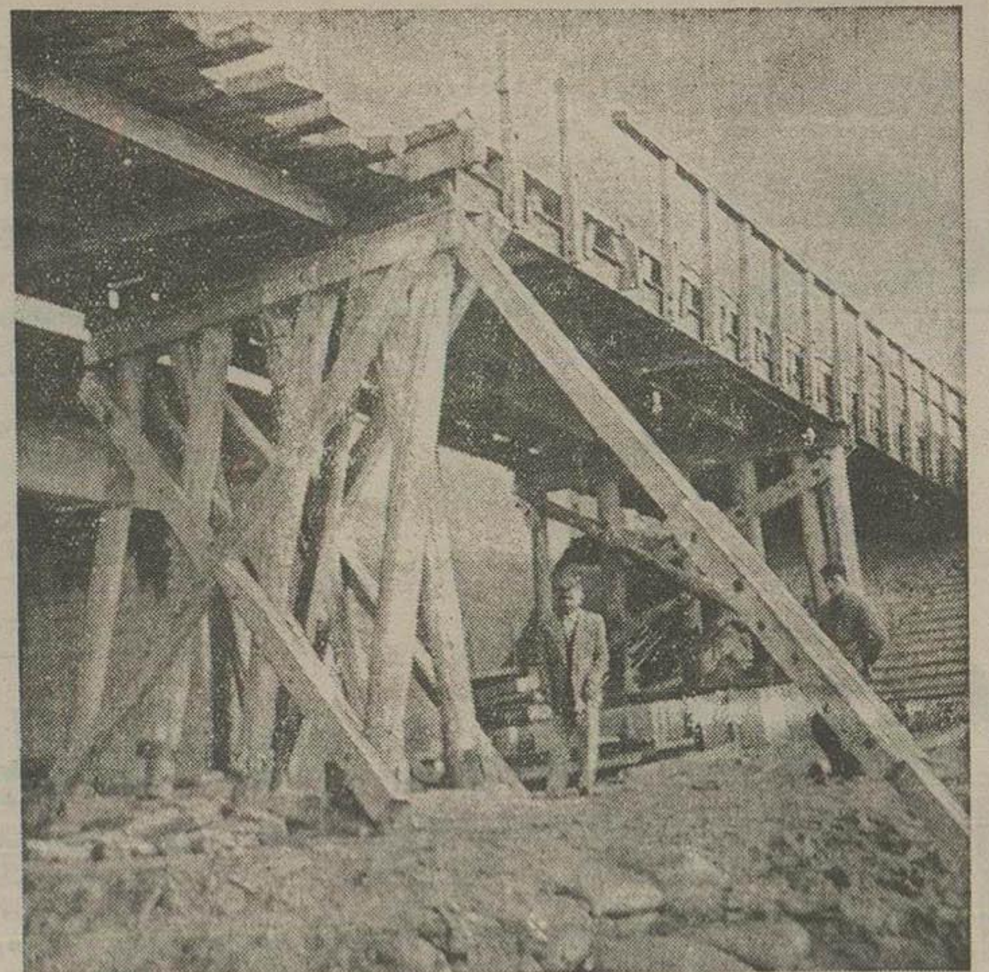
در این عکس قسمتی از پل غازیان که در دست تعمیر است دیده میشود
