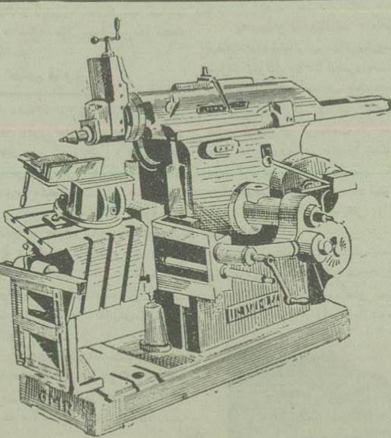
معروفترین ماشینهای صفحه تراش ساخت کارخانه معروف انگلیسی
