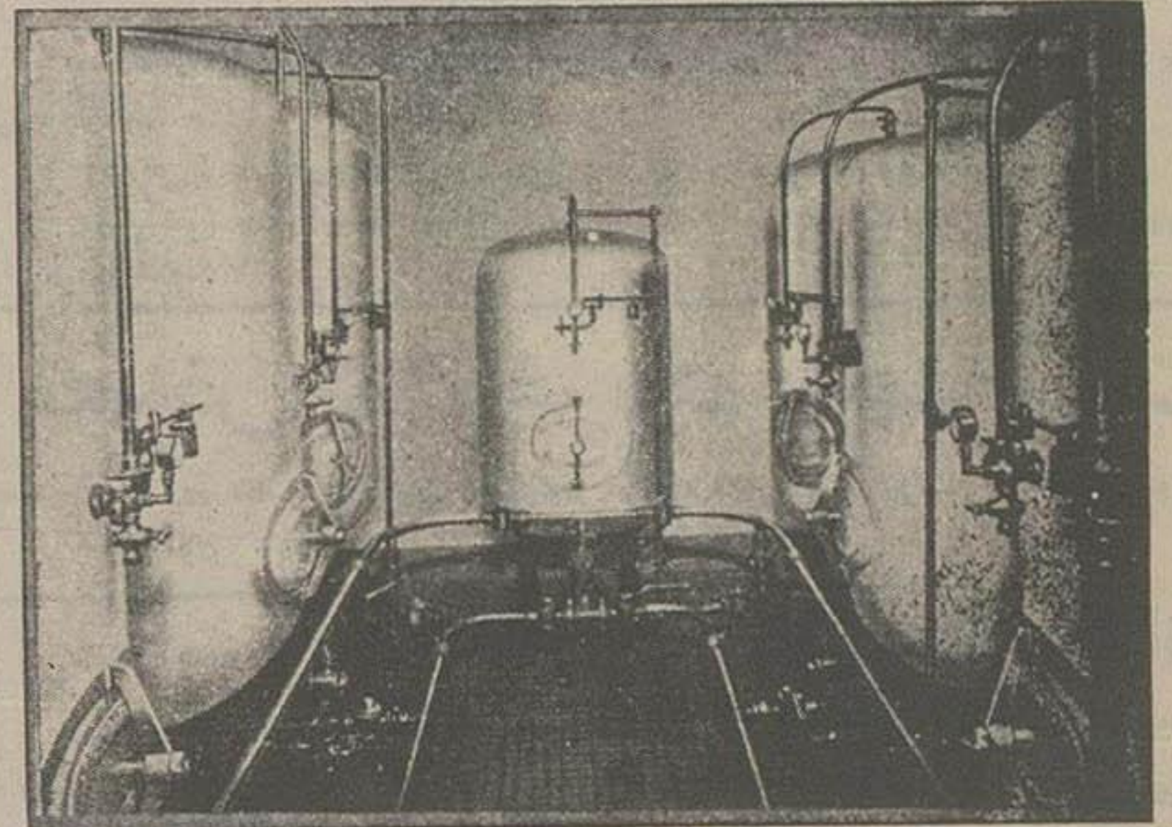
یک منظره از ماشین آلات کارخانه آبیو سازی ساهاکیان تبریز
