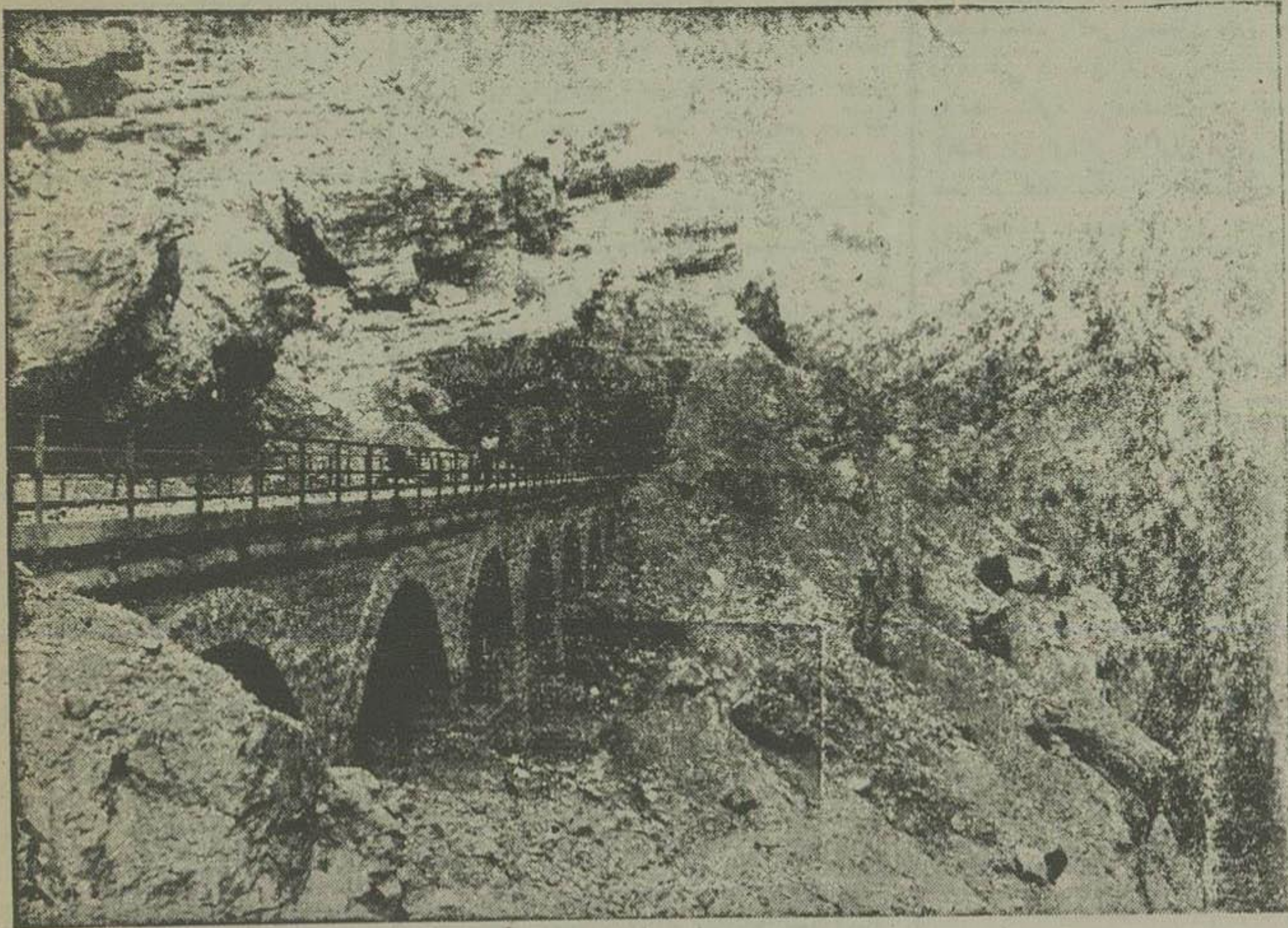
در این کاشه مدخل یکی از تونل های خط آهن جنوب و و بادوکی که پیش از رسیدن به تونل در یکی از دره های شمال دزفول ساخته شده بنظر میرسد
