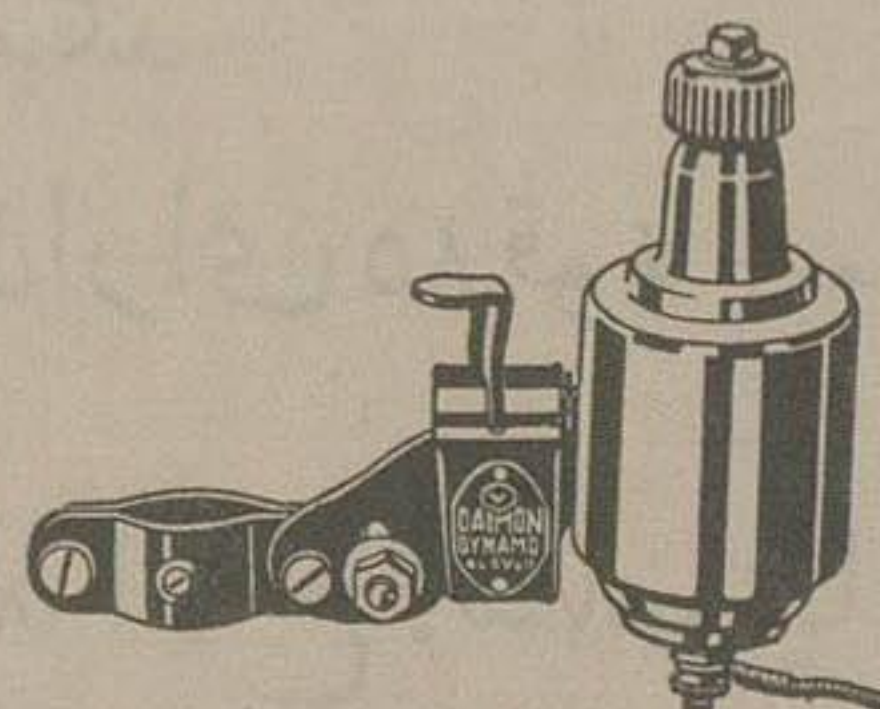
دینام برای دو چرخه قوه شش ولت
