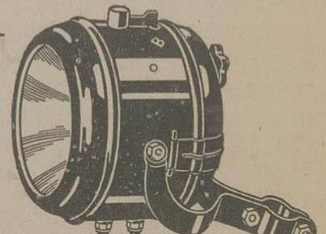
چراغ جلو دو چرخه که علاوه بر سوزن بوسیله دینام محل قوه و لامپ یک کی را دار است
