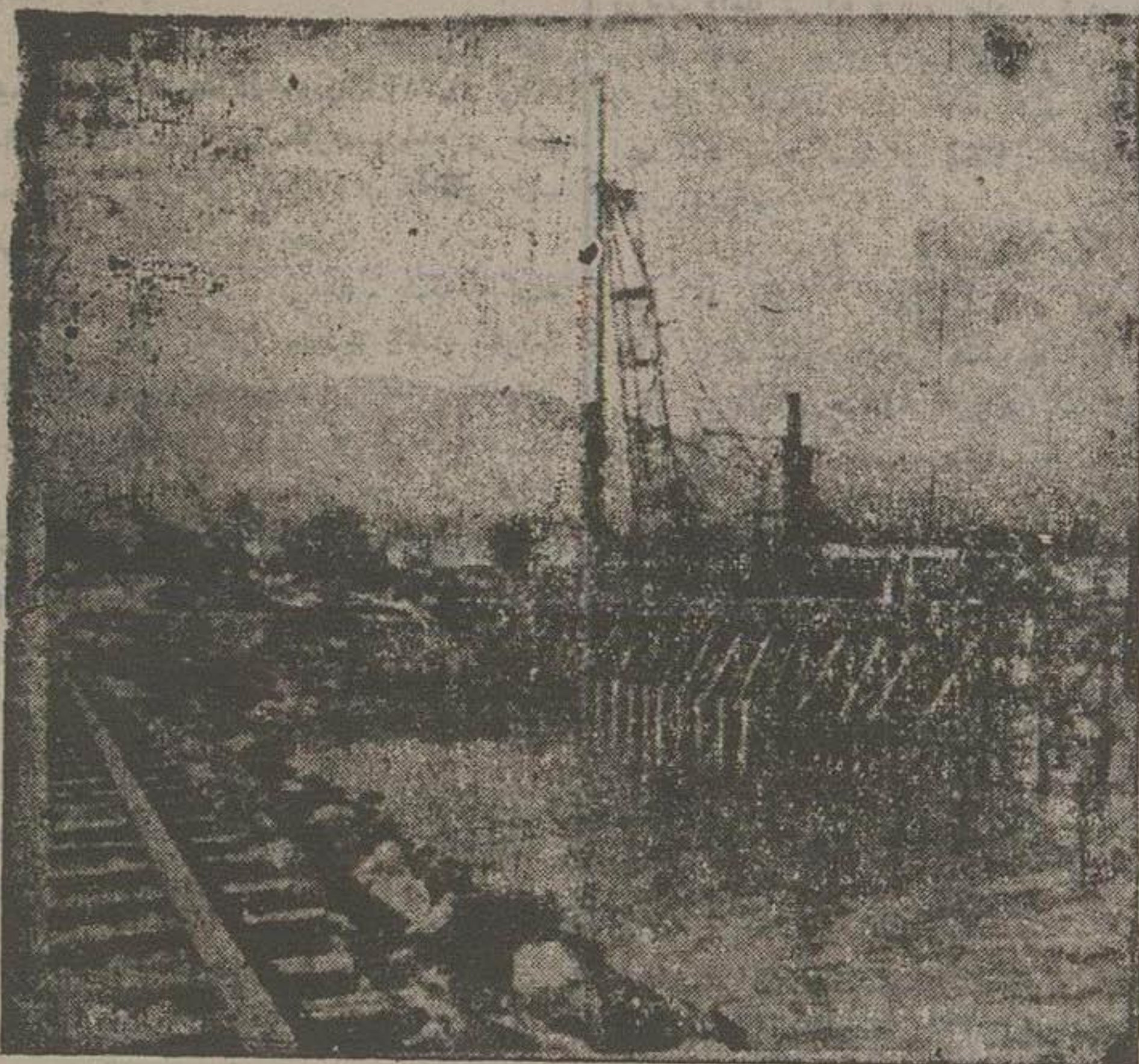
منظره از عملیات ساختمانی موج شکن شماره ۴ بندر نوشهر هنگامی که چکش بختری مشغول کوبیدن دبل (لارس) های آهنی کنار آن در دریا میباشد
