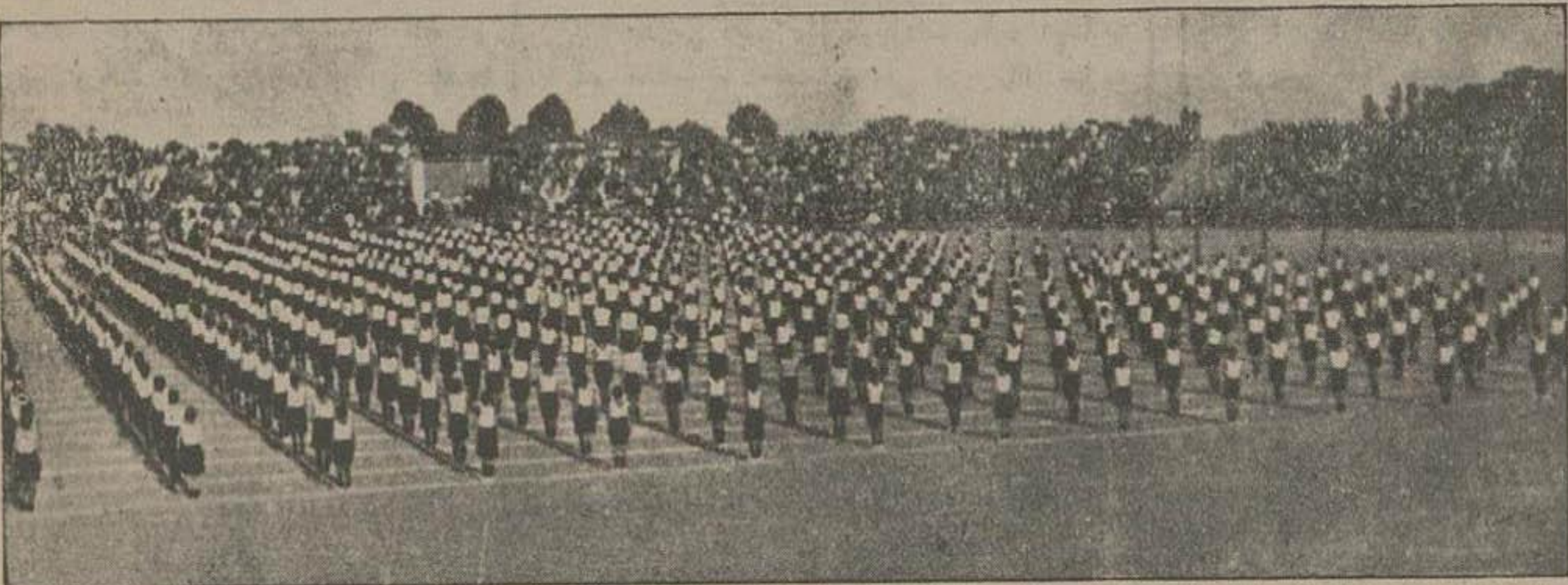
دو هزار نفر محصل جوان در میدان امجدیه نمایشات ورزشی دادند ان ورزشکاران خورد - ال چندین قسم ورزشهای بدنی و تفریحی را با آمک موزیک بطرز بسیار جالب توجهی انجام دادند
