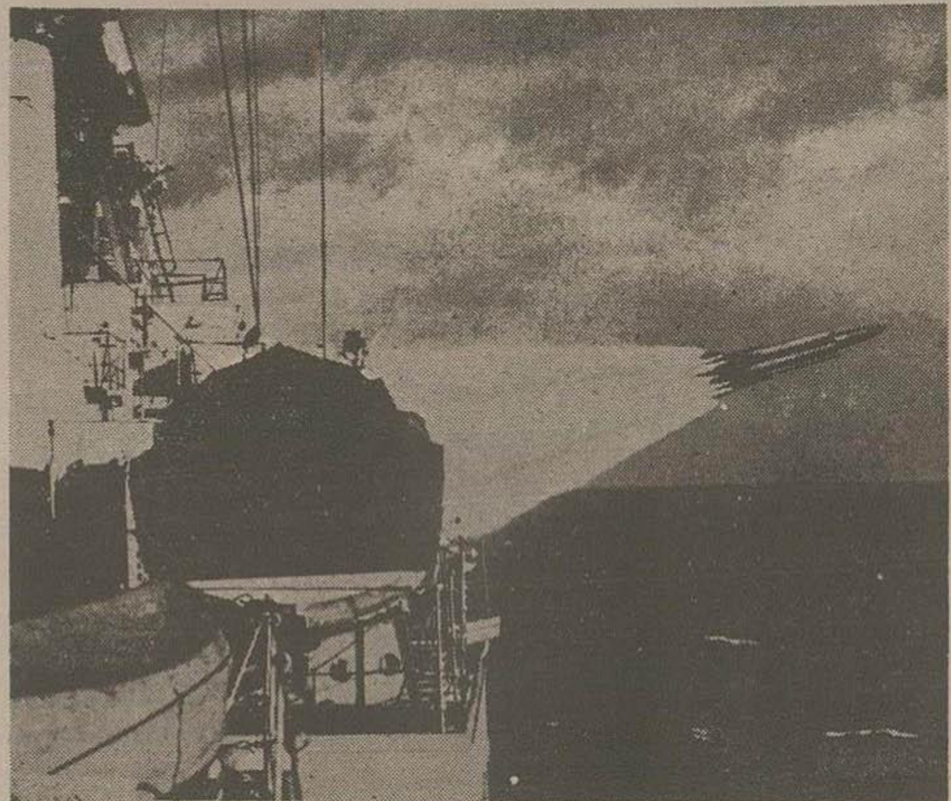
موشک هدایت شونده می اسلاک هنگامیکه تاب از کشتی موشک انداز آزمایشی نیروی دریائی انگلیس این موشک بر ضد هواپیما مکرر می رود و هدف خود را باردار پیدا میکند.
