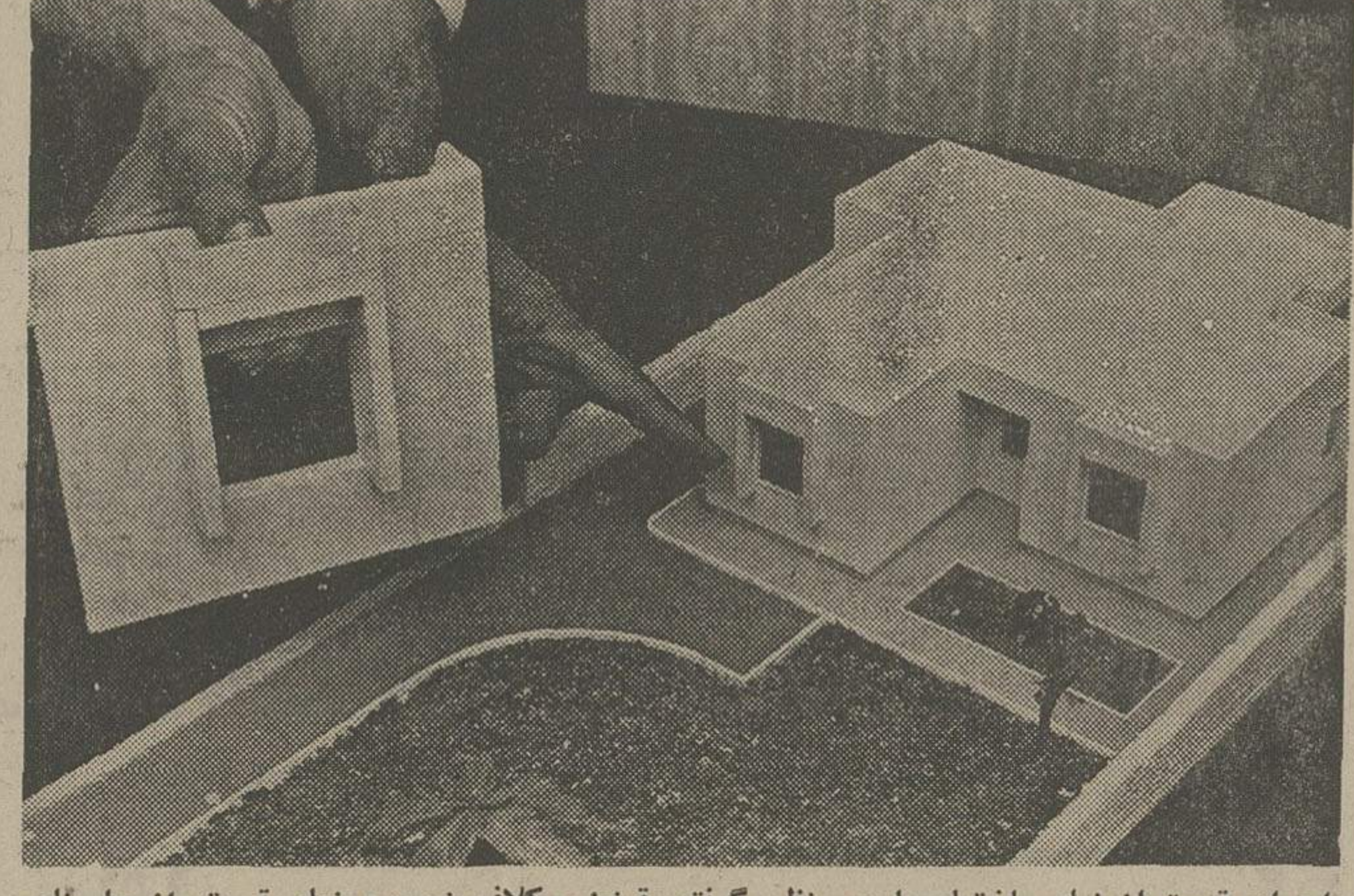
اجرای قسمتی از نمای ساختمان با در نظر گرفتن قرینز و کلاف پنجره و نمای قسمتی از جانب پناه.
